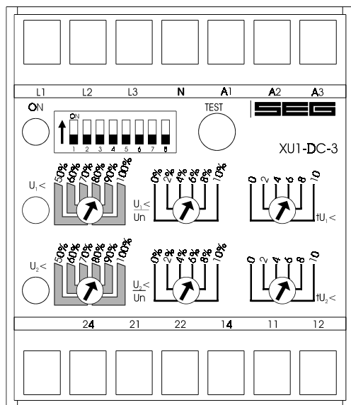
Fig. 4.2: Front plate XU1-DC-3
